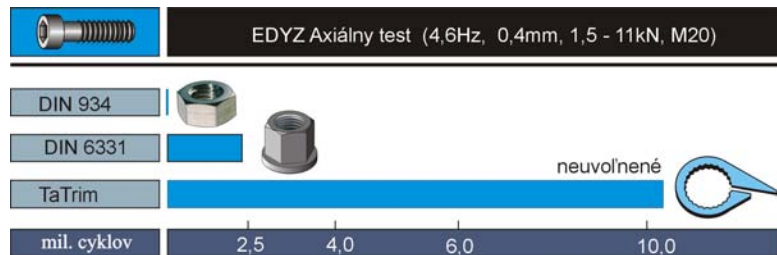
Obr. 2 Vibračný test EDYZ
